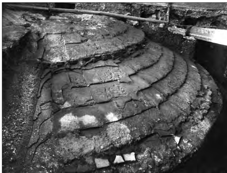
Fig. 5. Il sistema di copertura dell'estradosso della volta dell'aula del Piccolo Emiciclo.
